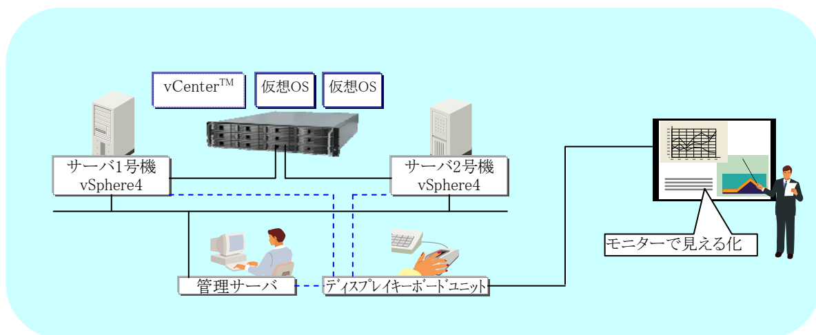
図1. VMware vSphere™仮想化デモンストレーション構成の例
